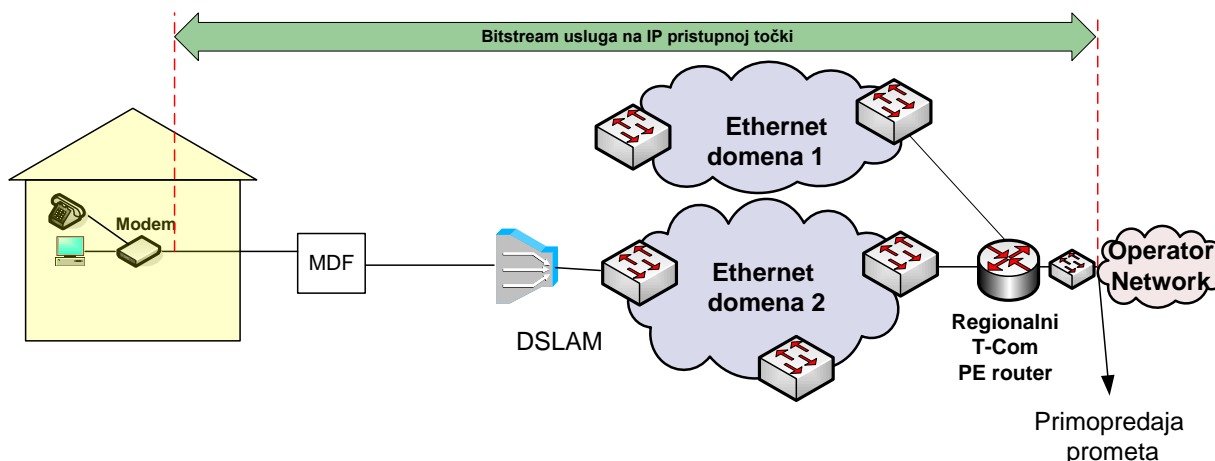
Slika 13. Veleprodajni širokopolasni pristup za pružanje VoIP usluge na IP razini u slučaju kada Krajnji korisnik ostvaruje Osnovni pristup mreži putem usluge Operatora korisnika
