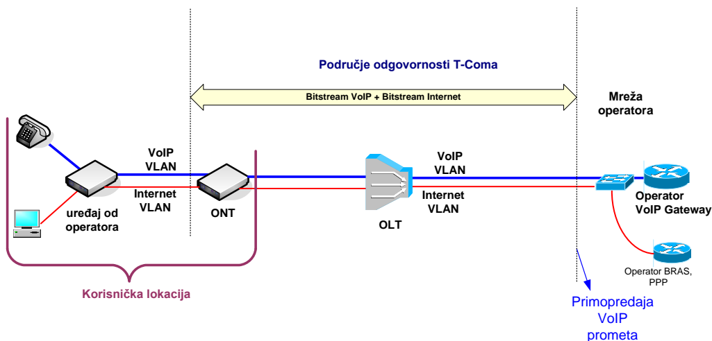
Slika 14. Veleprodajni širokopolasni pristup za pružanje VoIP usluge preko FTTH pristupa (GPON) na OLT razini
